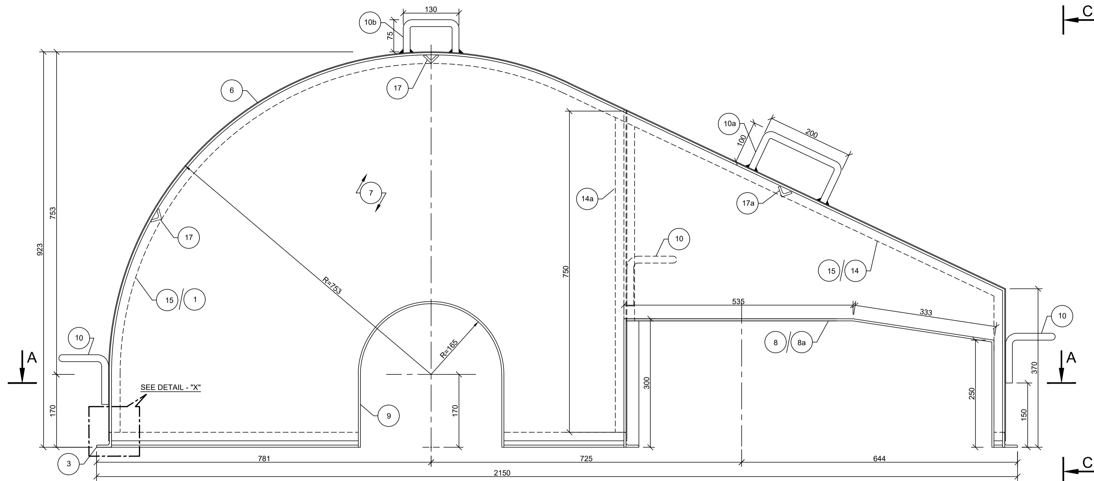
ELEVATION
