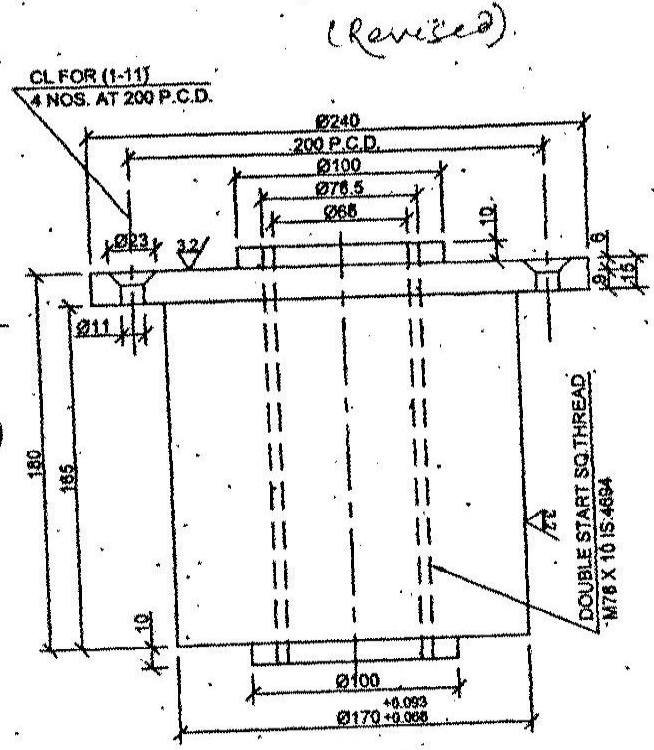
ELEVATION
